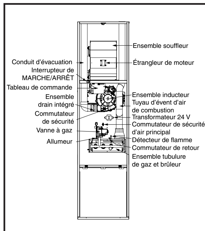
Figure 23. Composants de la fournaise
