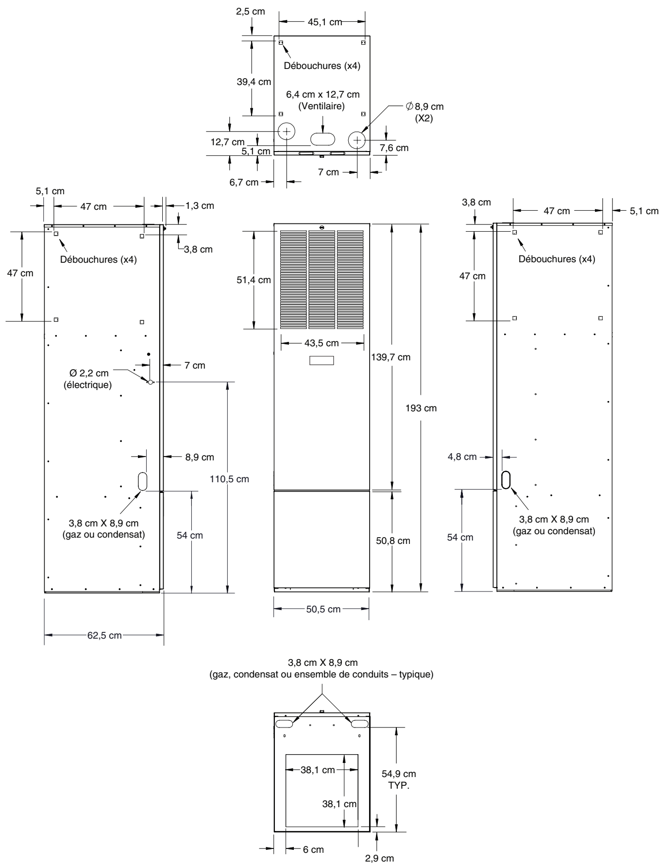
Figure 25. Reprise avant sur les armoires (avec boîtier de serpentin) (boîtiers de retour qui se terminent par ABM)
