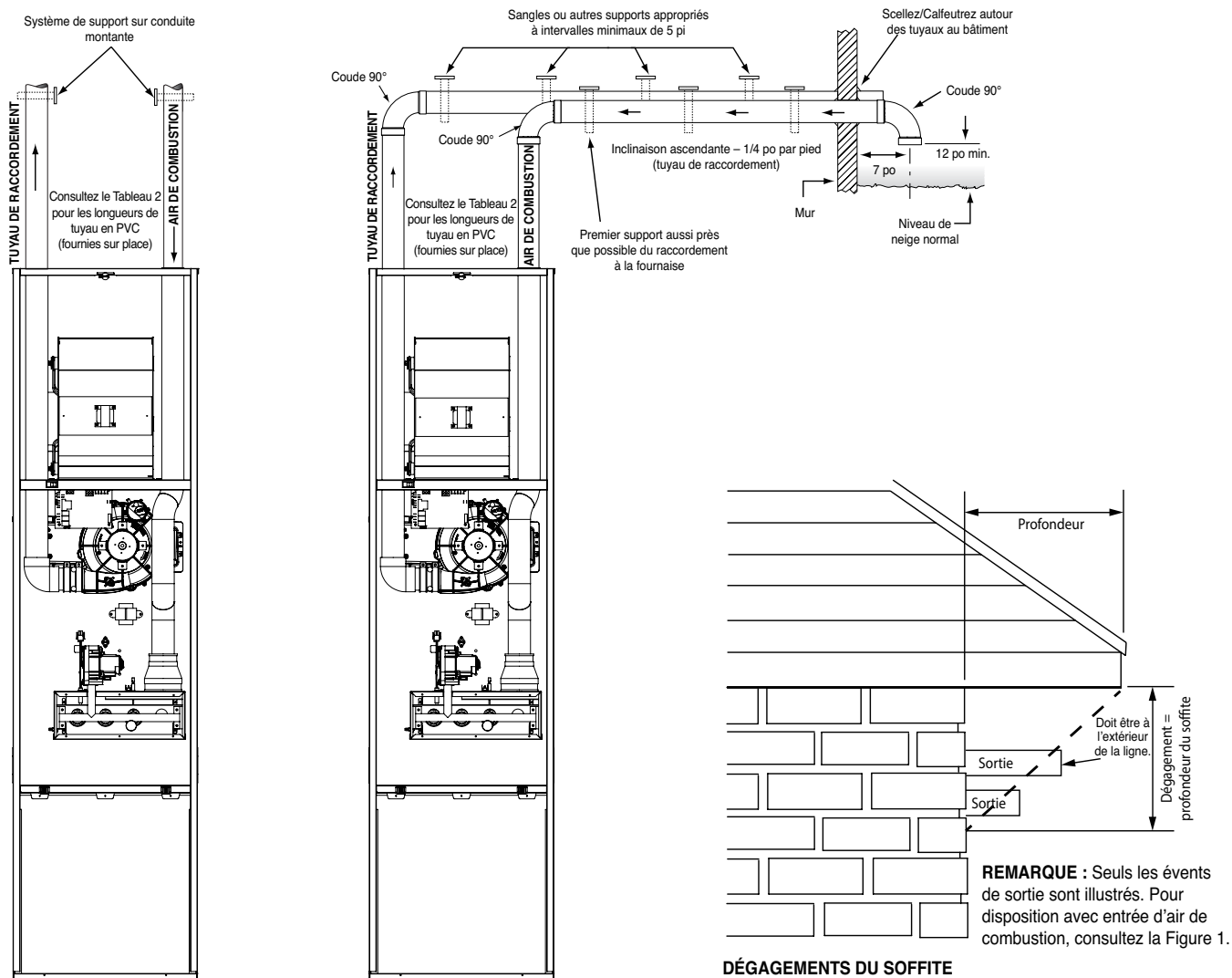
Figure 36. Évacuation horizontale/verticale et dégagements au soffite
