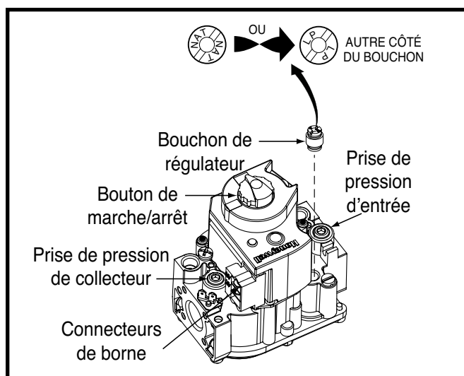
Figure 20. Robinet de gaz
