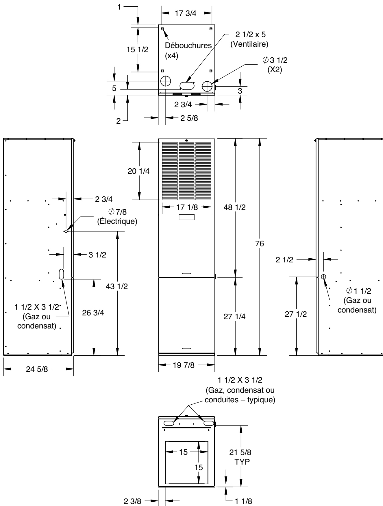
Figure 28. Armoires à reprise d'air avant (avec boîtier de serpentin) (armoires à reprise d'air avec le suffixe ACM)
