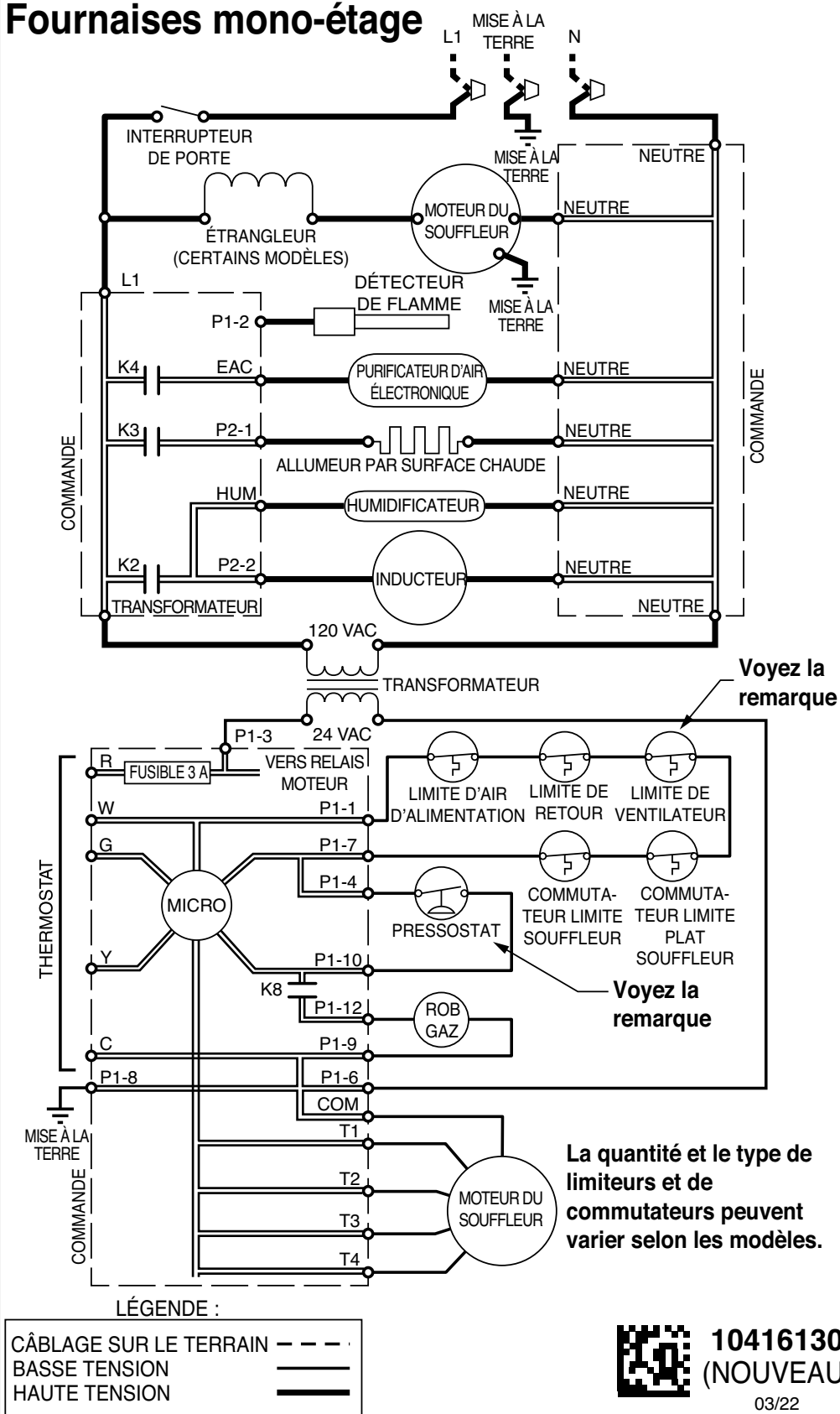
Figure 35. Schéma à contacts Emerson
