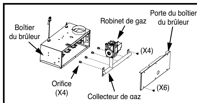
Figure 21. Démontage de l'orifice
