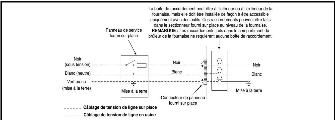
Figure 22. Câblage d'excitation de tension de ligne
