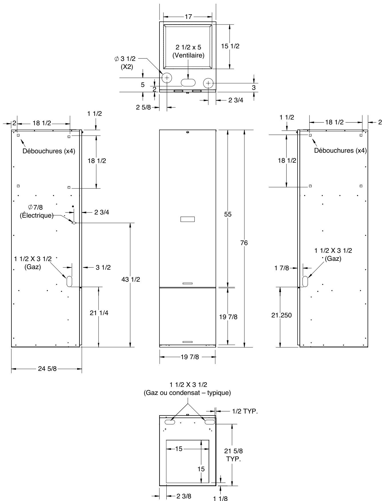
Figure 30. Armoires de reprise d'air par le haut (avec boîtier de serpentin) (armoires de reprise d'air avec le suffixe ABM)
