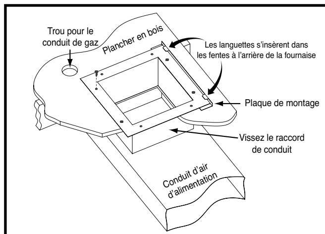
Figure 15. Conduits d'air étroits – Option 2
