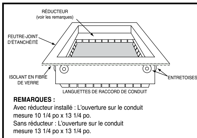
Figure 9. Raccord de conduit
