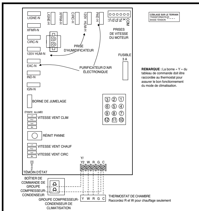
Figure 24. Câblage sur terrain Emerson, quatre fils, applications de chauffage/ climatisation
