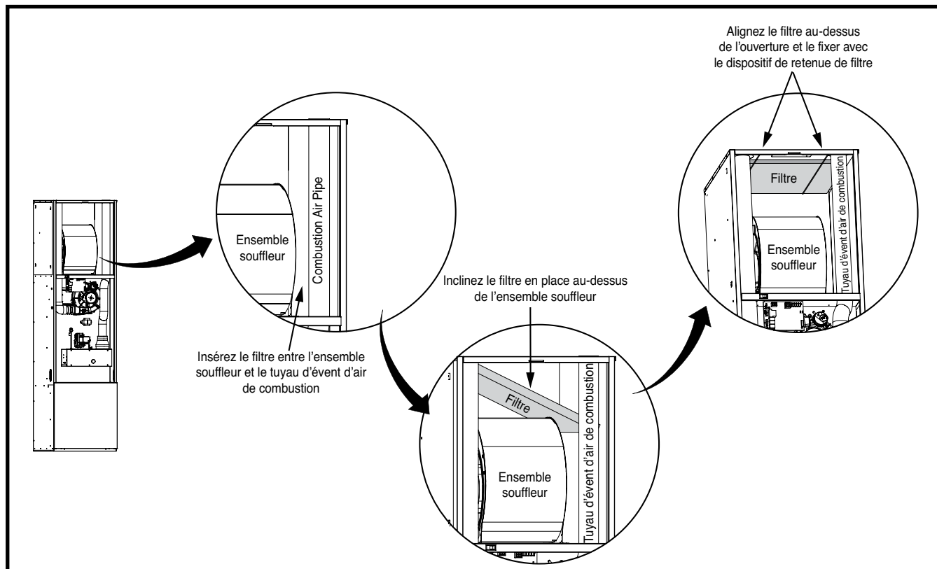
Figure 8. Installation du filtre
