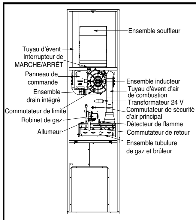
Figure 25. Composants de la fournaise
