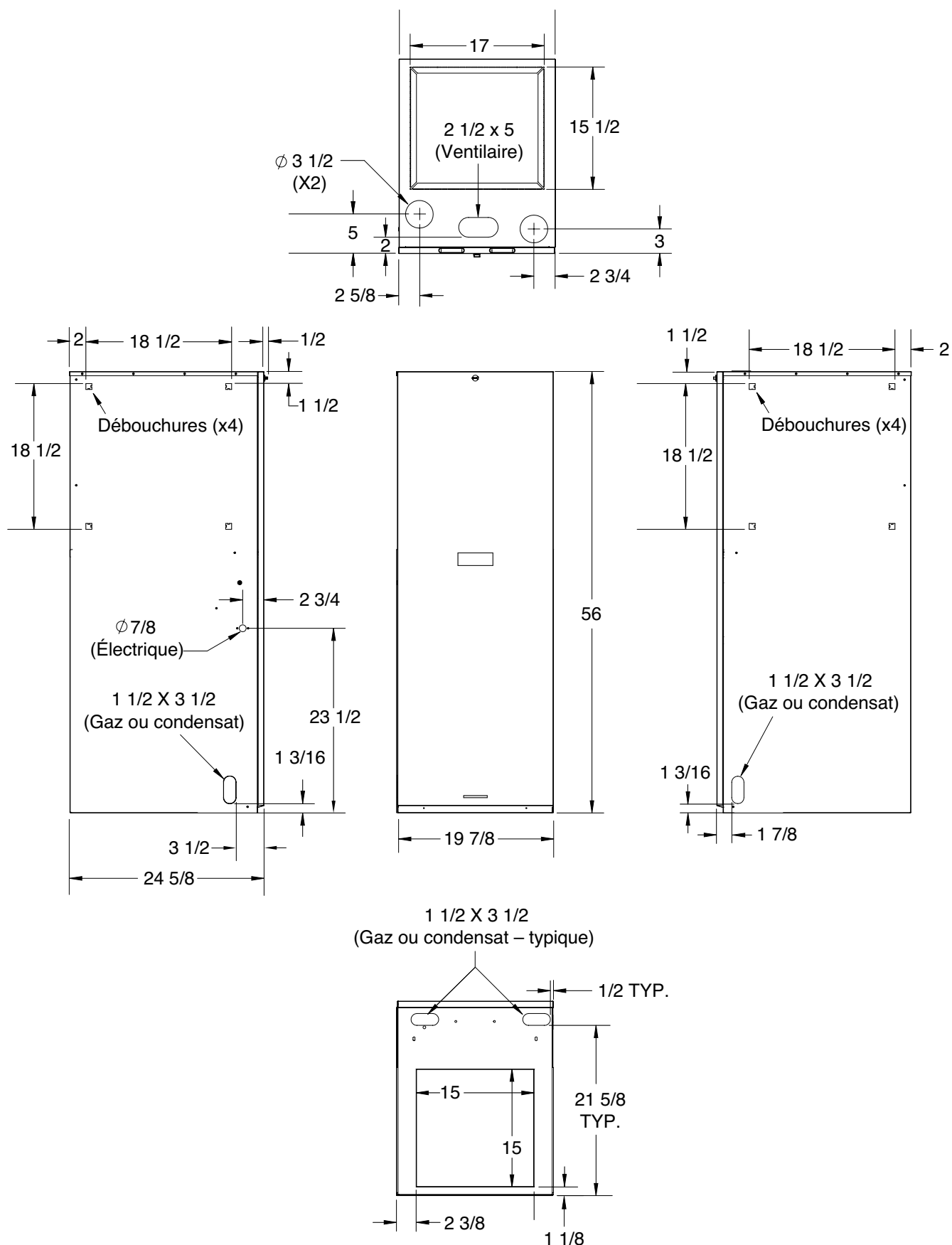
Figure 29. Armoires de reprise d'air par le haut (sans boîtier de serpentin)
