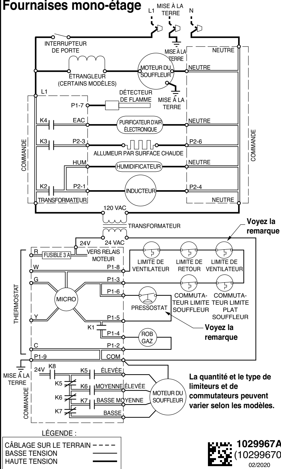
Figure 34. Schéma à contacts Nordyne/UTEC
