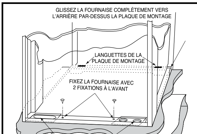
Figure 17. Fournaise de placard sur conduit d'air d'alimentation
