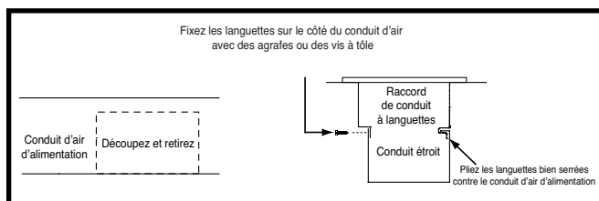
Figure 14. Conduits d'air étroits – Option 1
