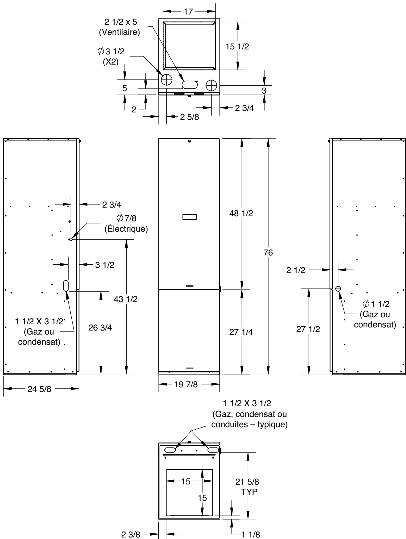
Figure 31. Armoires de reprise d'air par le haut (avec boîtier de serpentin) (armoires de reprise d'air avec le suffixe ACM)
