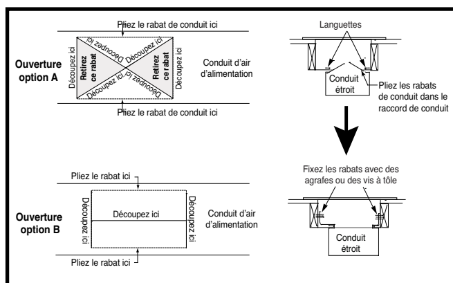
Figure 13. Raccord de conduit à vis
