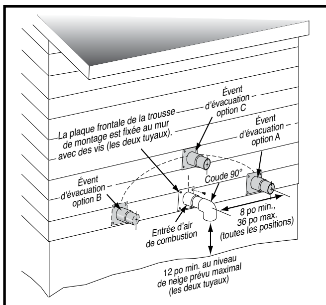
Figure 1. Dégagements du tuyau d'admission et du tuyau d'évacuation
