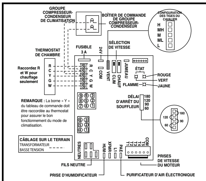
Figure 23. Excitation de tension de ligne, quatre fils Applications d chauffage/climatisation
