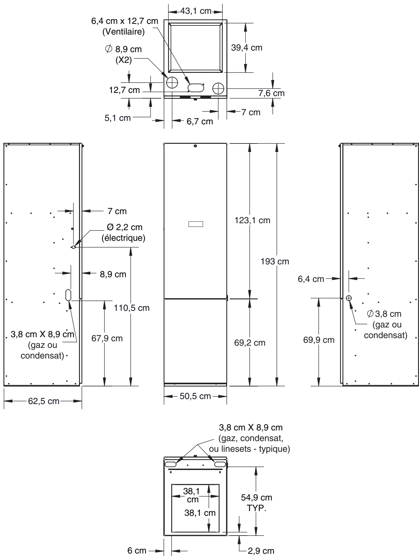
Figure 29. Retour supérieur sur les armoires (avec boîtier de serpent) (boîtiers de retour qui se terminent par ACM)
