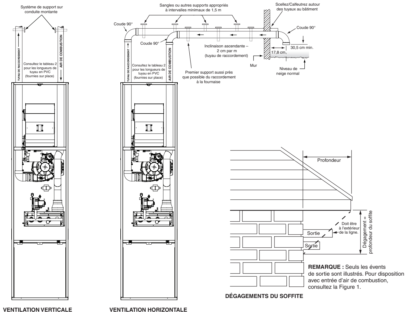
Figure 34. Évacuation horizontale/verticale et dégagements du soffite
