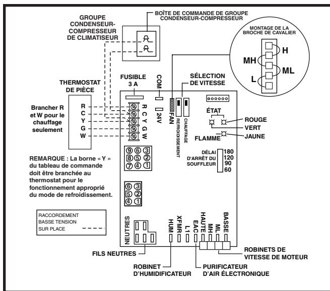
Figure 22. Applications de chauffage/climatisation, quatre fils, basse tension, sur le terrain Nordyne/UTEC
