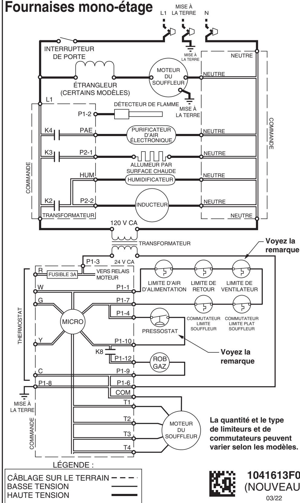
Figure 33. Schéma en échelle Emerson
