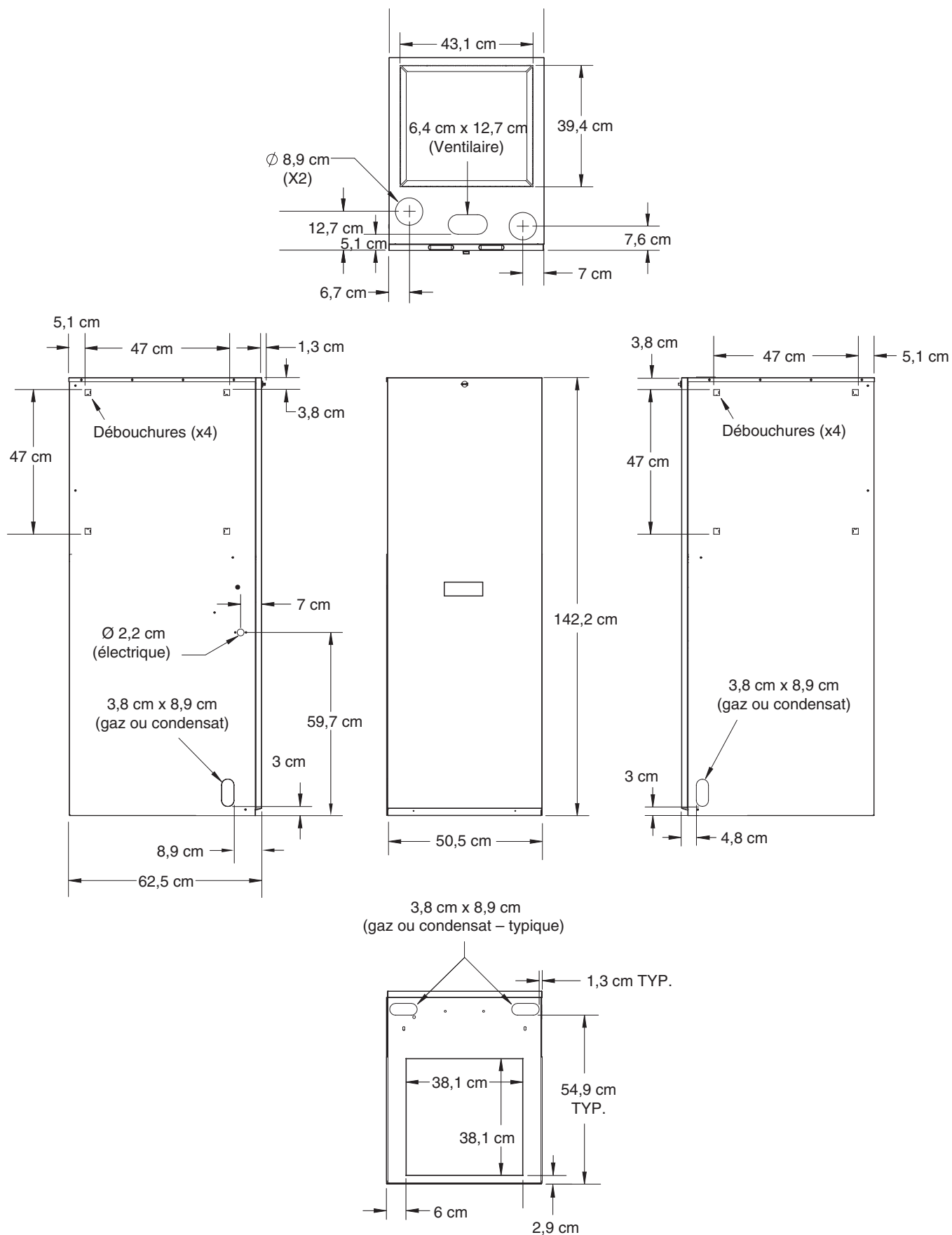
Figure 27. Retour supérieur sur les armoires (sans boîtier de serpent)
