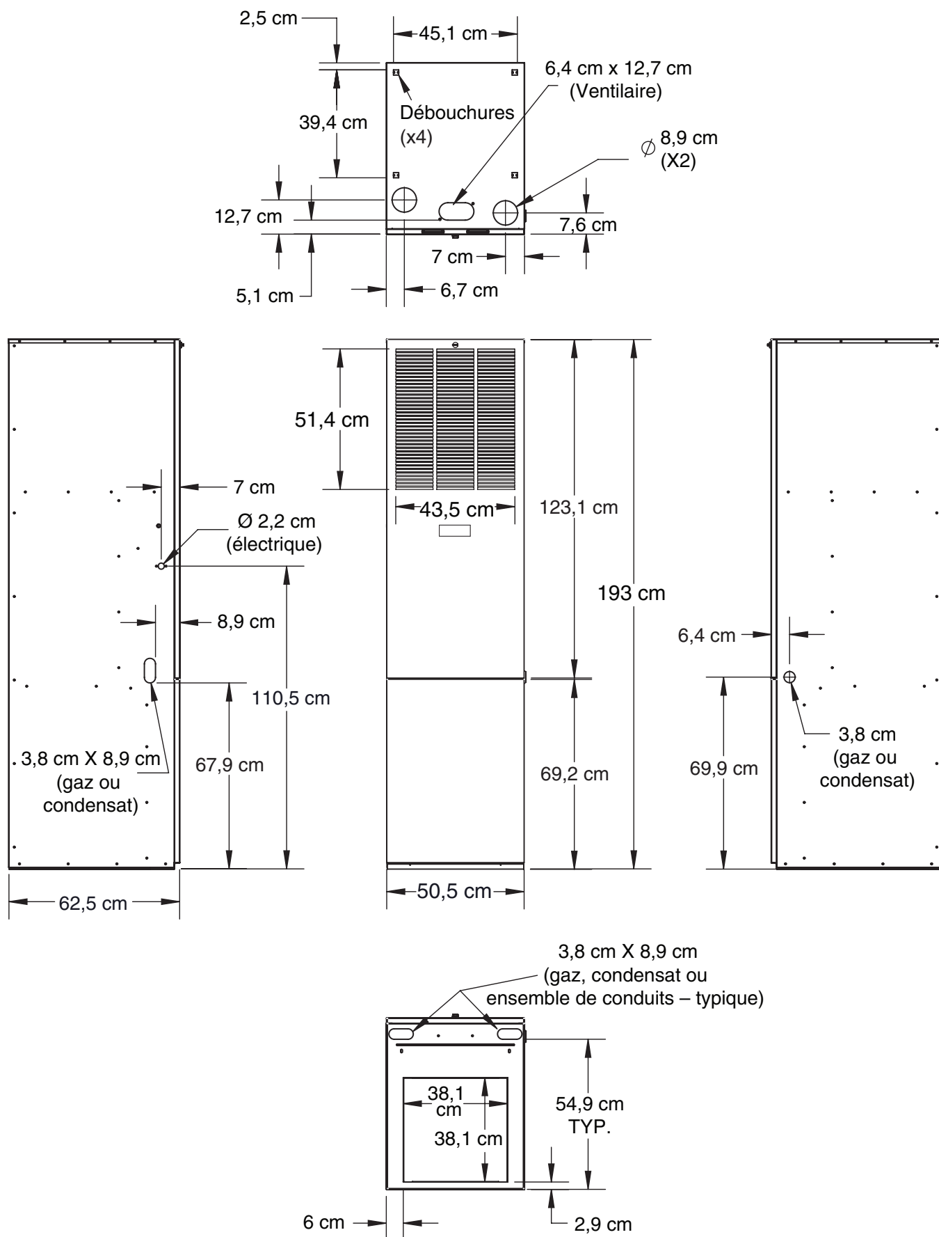
Figure 26. Reprise avant sur les armoires (avec boîtier de serpentin) (boîtiers de retour qui se terminent par ACM)
