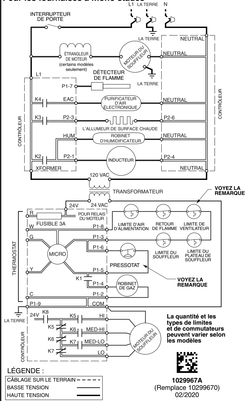
Figure 32. Schéma en échelle Nordyne/UTEC
