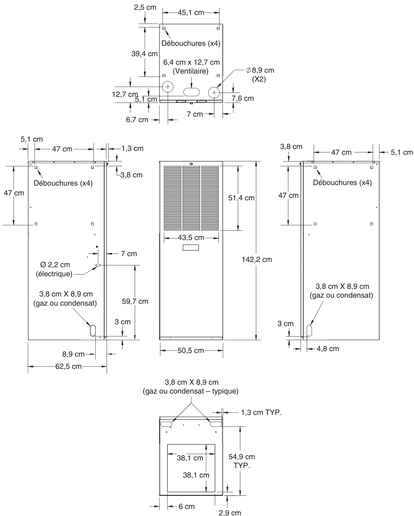
Figure 24. Reprise avant sur les armoires (sans boîtier de serpentin)
