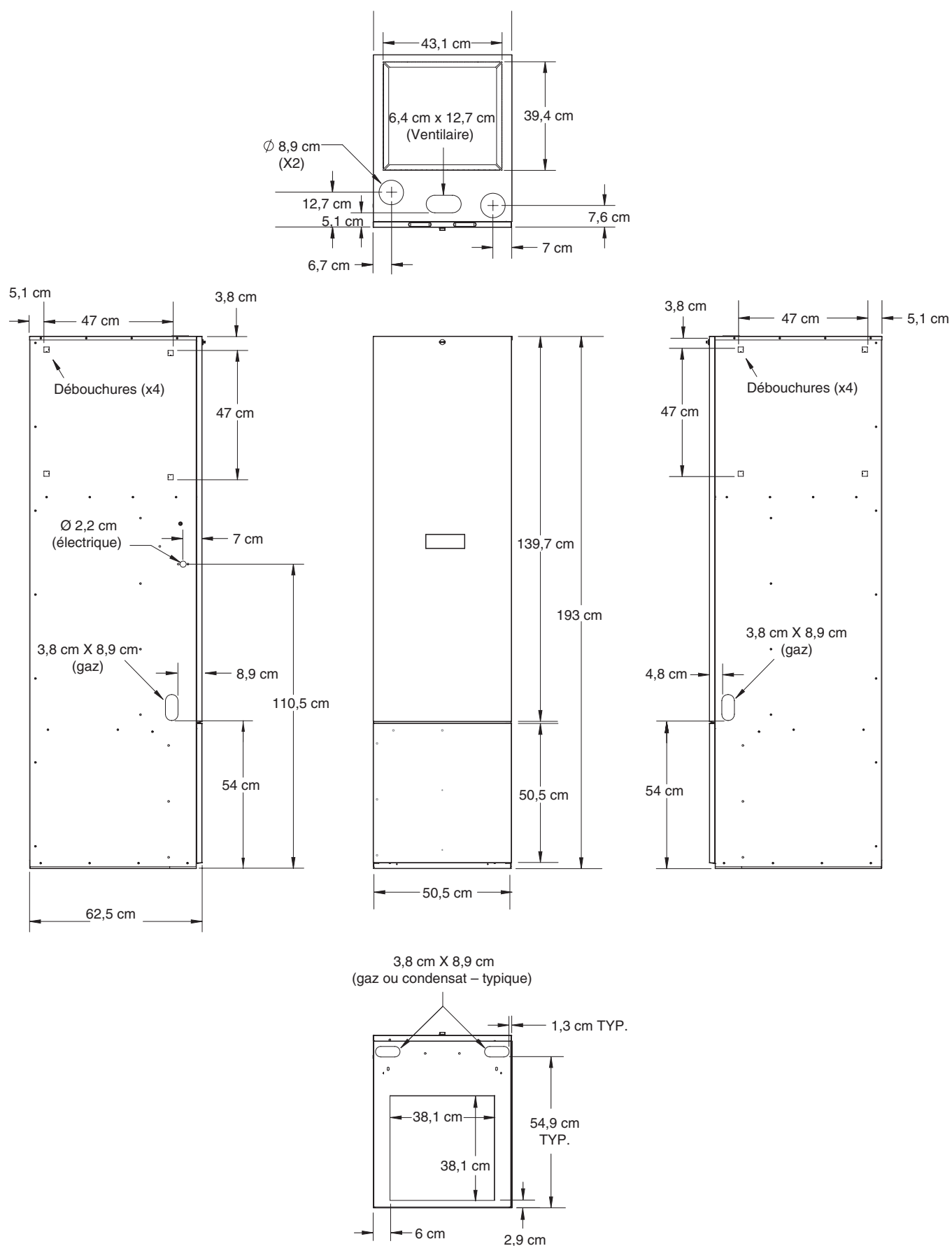
Figure 28. Retour supérieur sur les armoires (avec boîtier de serpentin) (boîtiers de retour qui se terminent par ABM)
