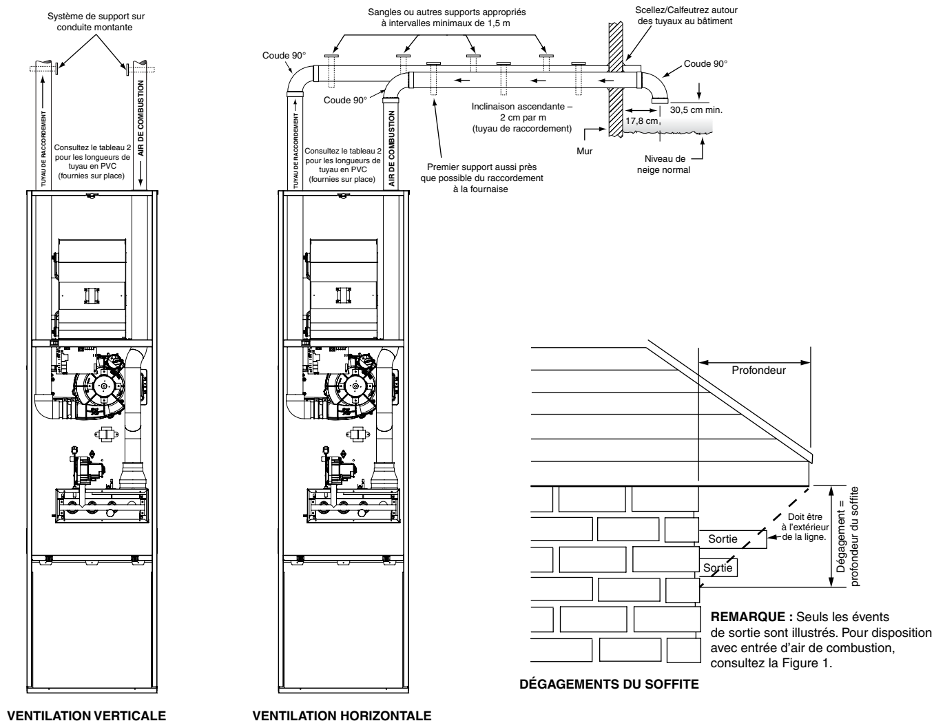
Figure 30. Évacuation horizontale/verticale et dégagements du soffite
