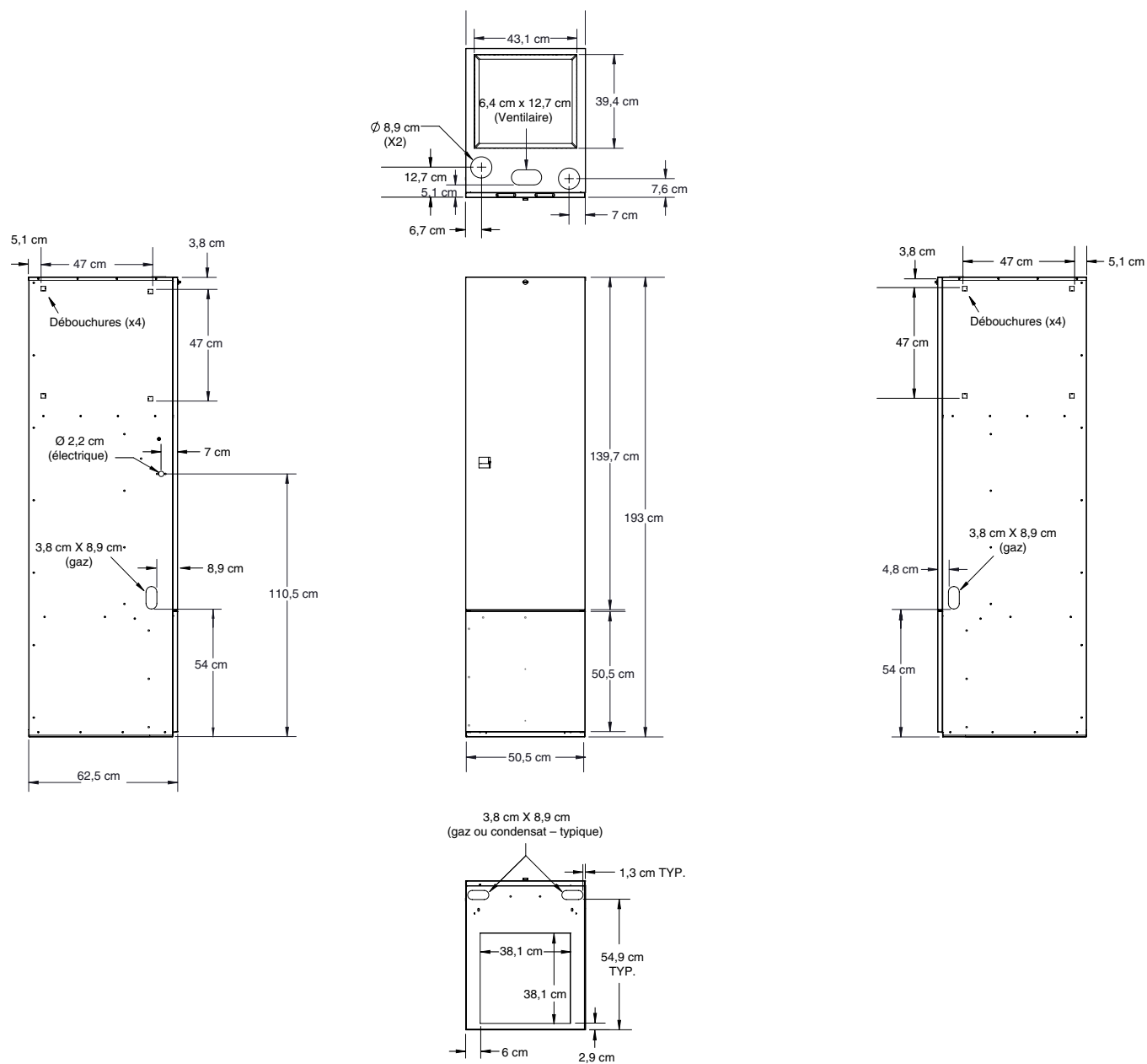
Figure 27. Retour supérieur sur les armoires (avec boîtier de serpentin)
