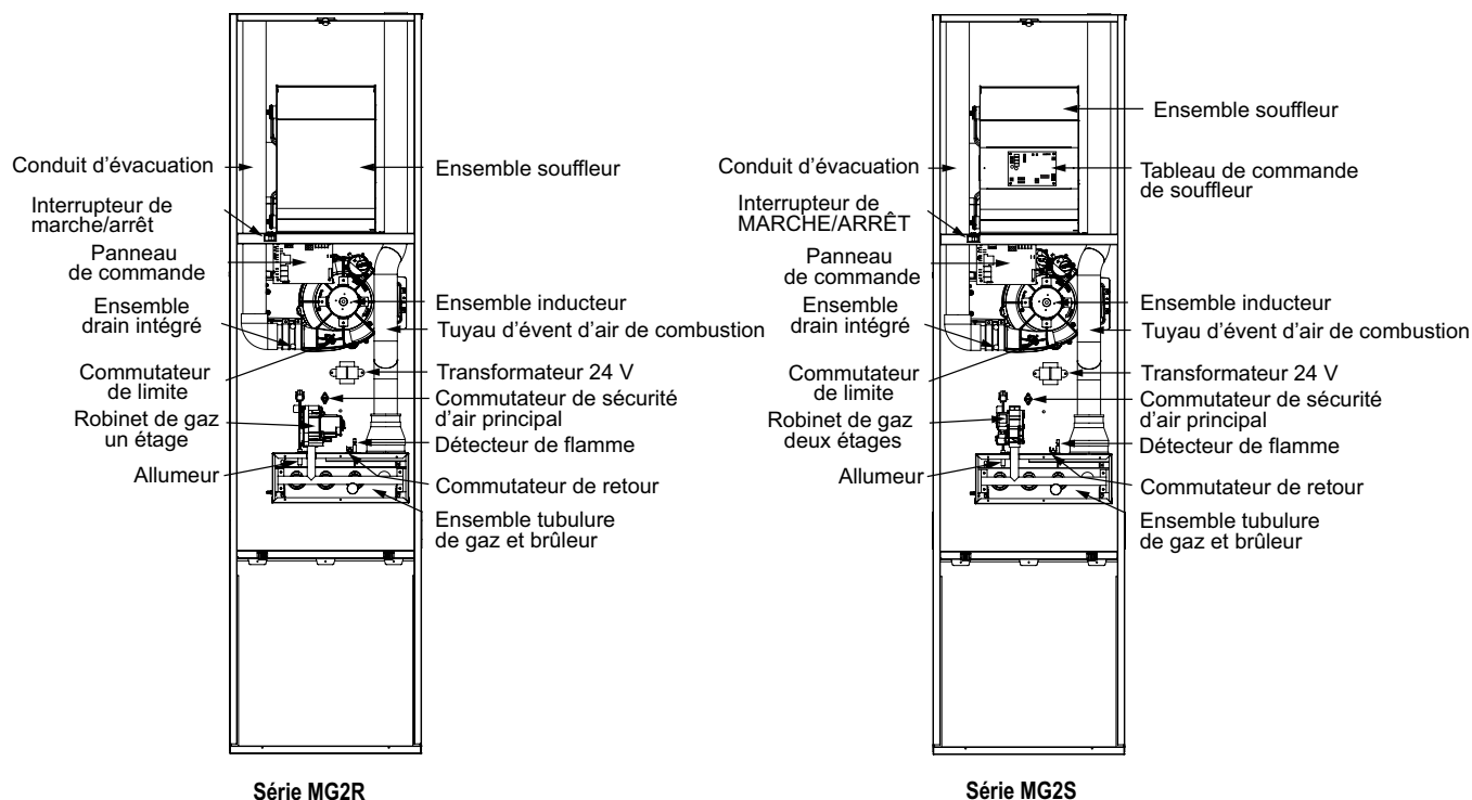
Figure 3. Composants des fournaies MG2R et MG2S
