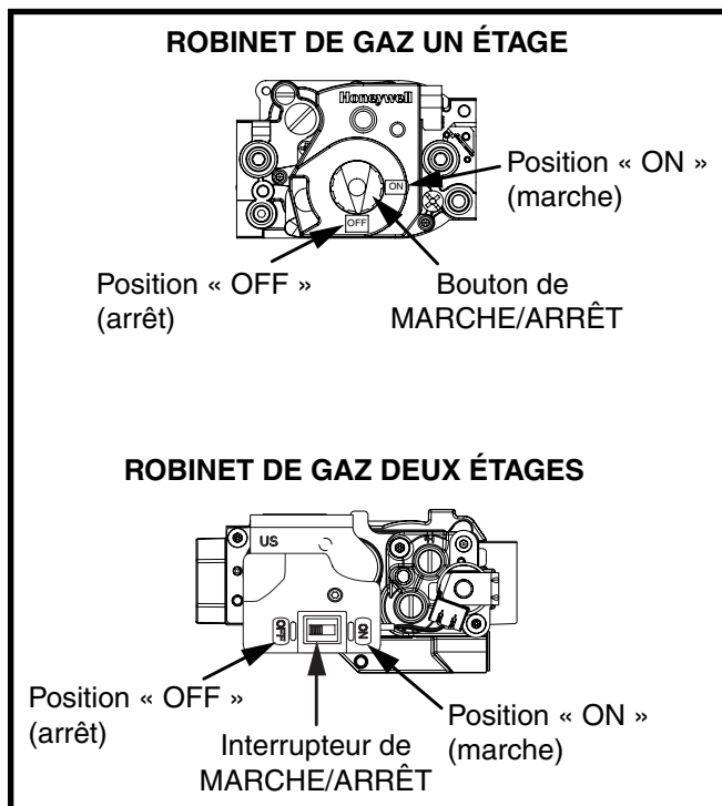
Figure 2. Vanne à gaz
