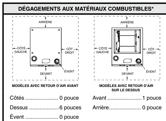
Figure 1. Dégagements minimaux
