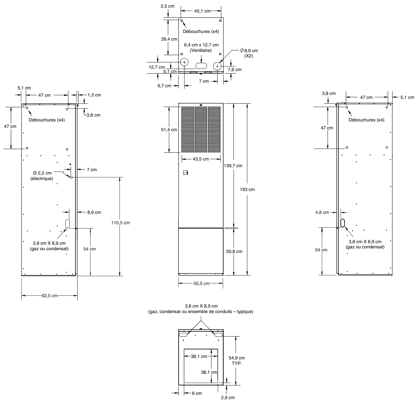
Figure 25. Reprise avant sur les armoires (avec boîtier de serpentin)
