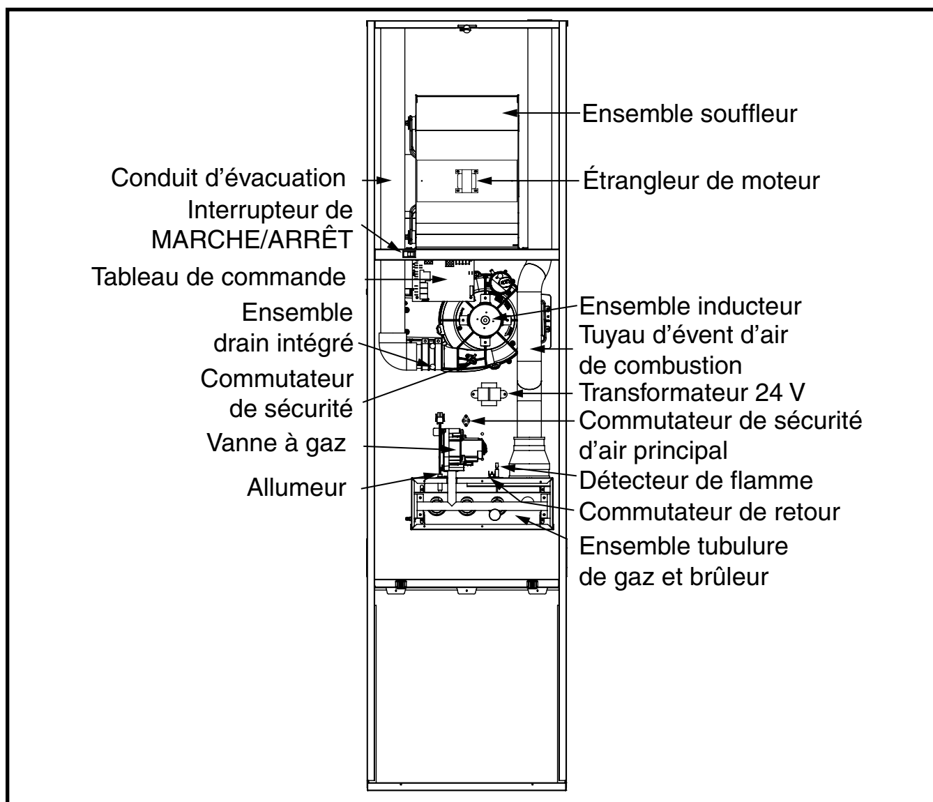
Figure 23. Composants de la fournaise
