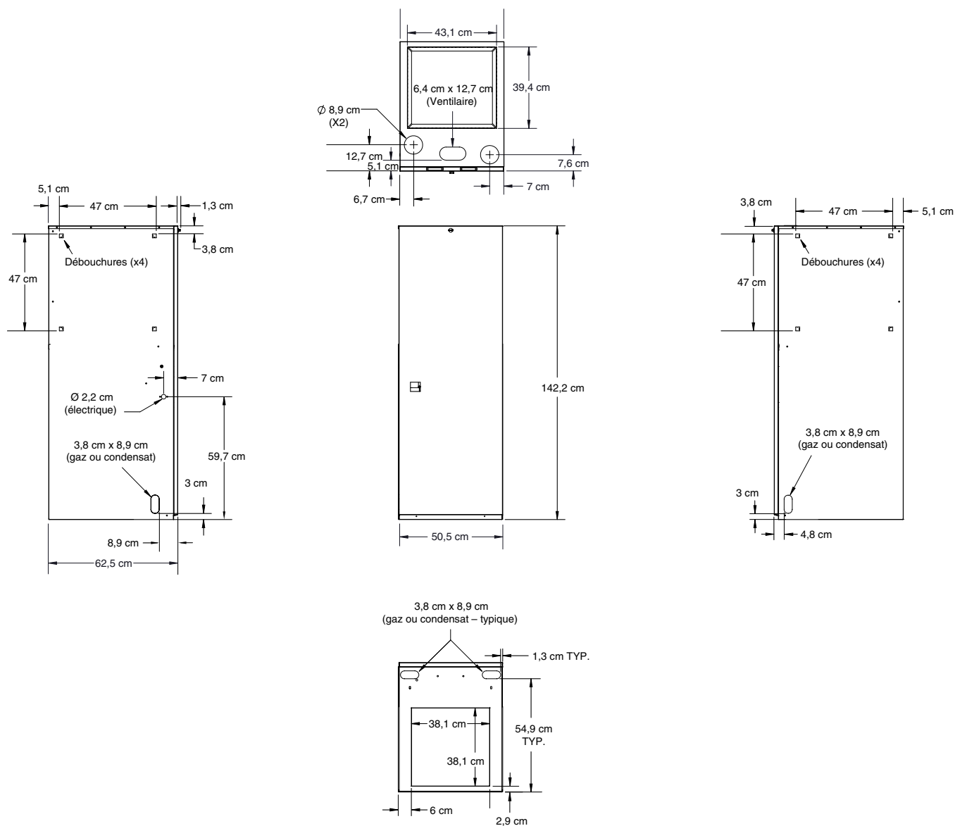
Figure 26. Retour supérieur sur les armoires (sans boîtier de serpent)
