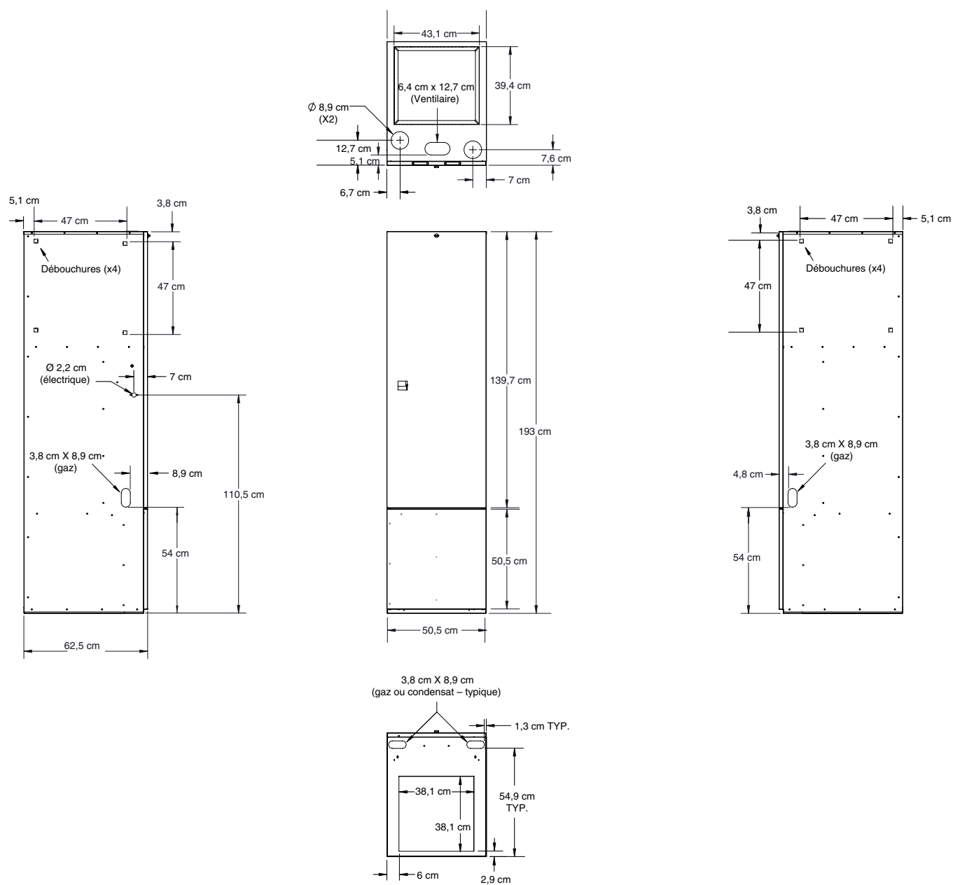
Figure 27. Retour supérieur sur les armoires (avec boîtier de serpentin)
