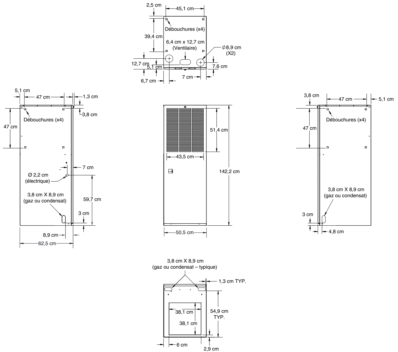
Figure 24. Reprise avant sur les armoires (sans boîtier de serpent)
