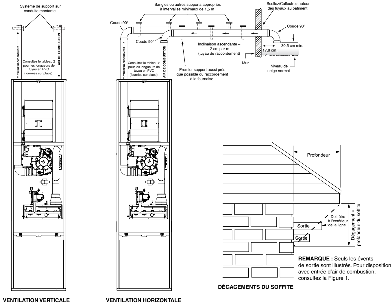
Figure 29. Évacuation horizontale/verticale et dégagements du soffite
