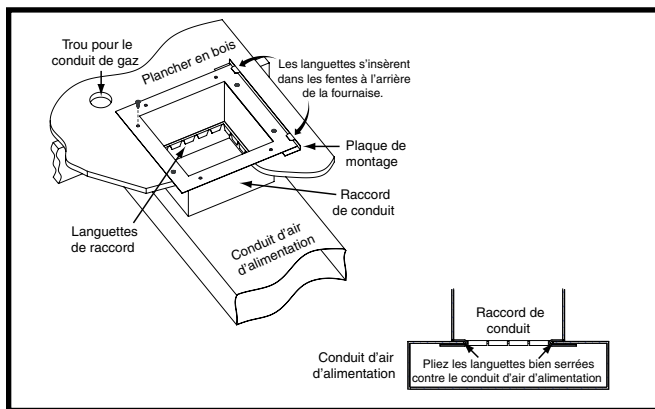
Figure 11. Raccord de conduit à languettes
