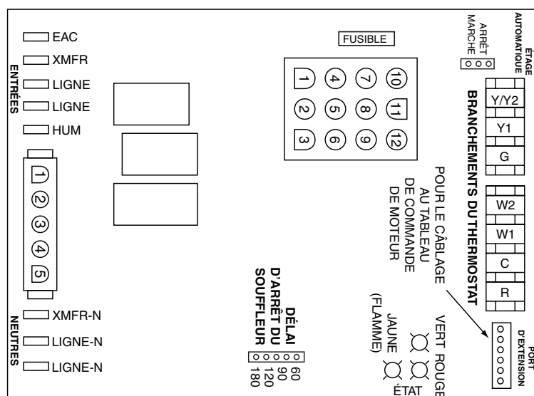
Figure 26. Tableau de commande de fournaise à deux étages
