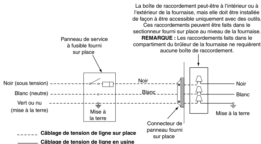
Figure 24. Câblage d'excitation de tension de ligne
