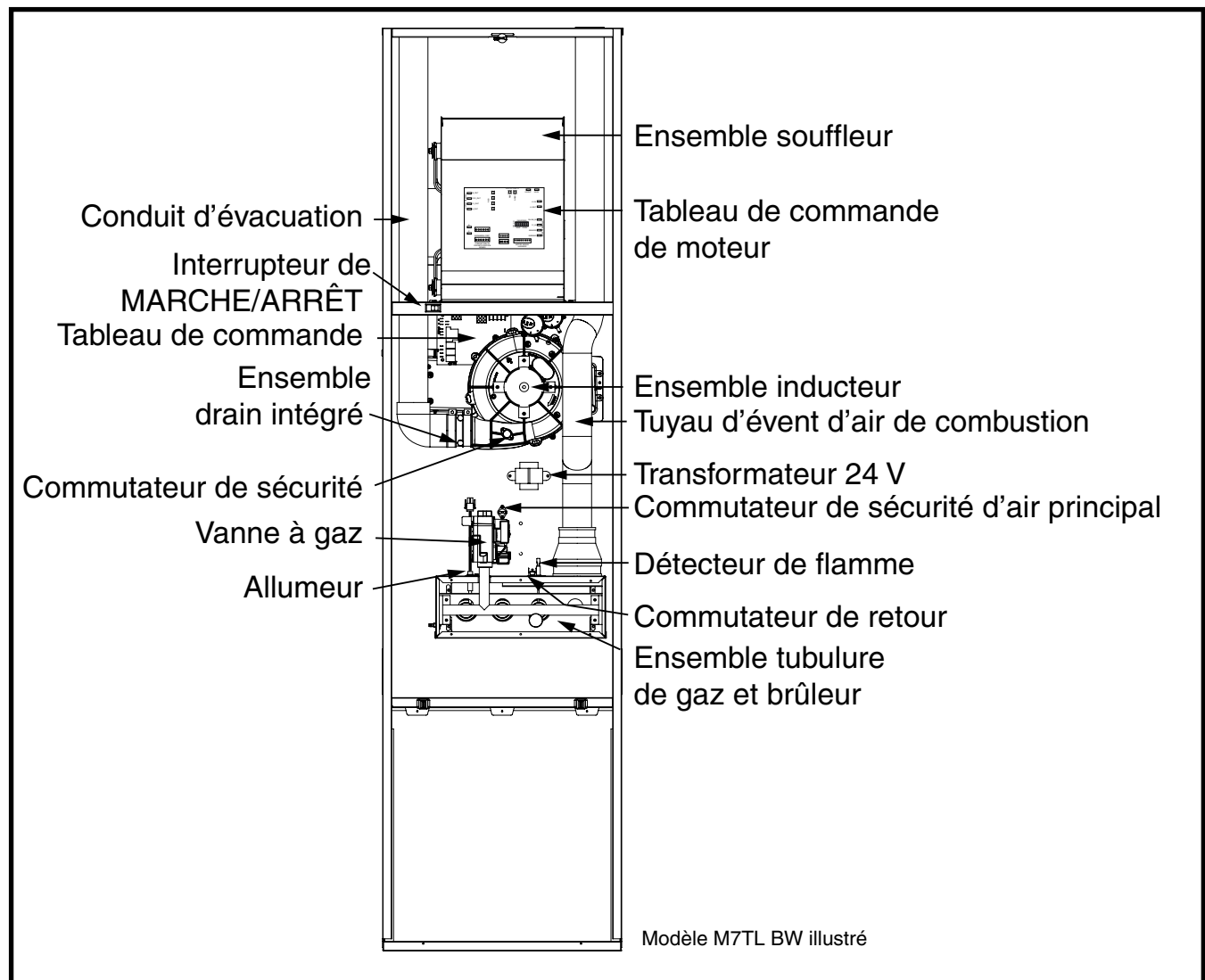
Figure 22. Composants de la fournaise
