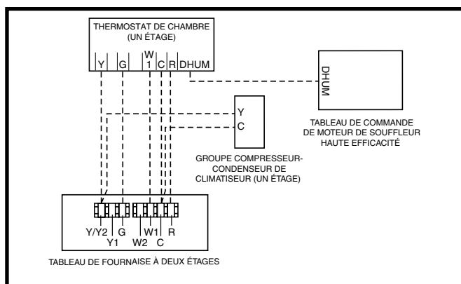
Figure 19. Configuration de câblage 1
