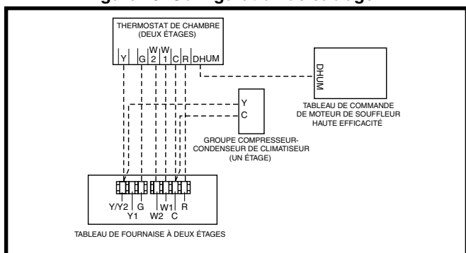
Figure 20. Configuration de câblage 2
