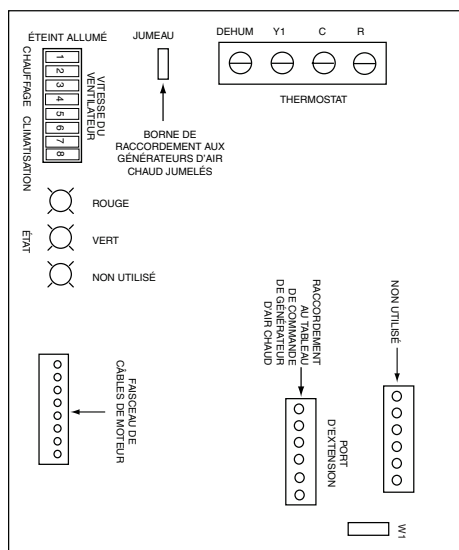
Figure 25. Tableau de commande de moteur MG2S
