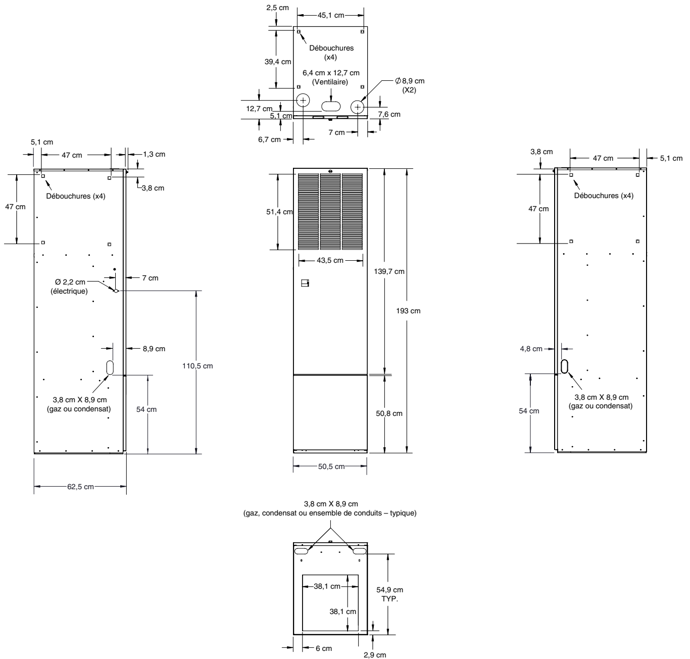
Figure 23. Avant modèle dimensions
