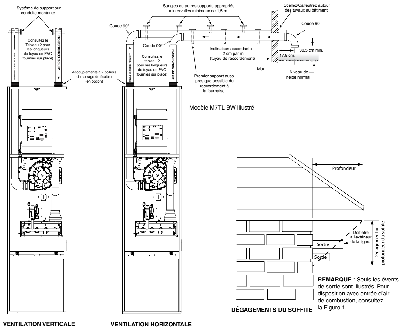
Figure 28. Évacuation horizontale/verticale et dégagements du soffite
