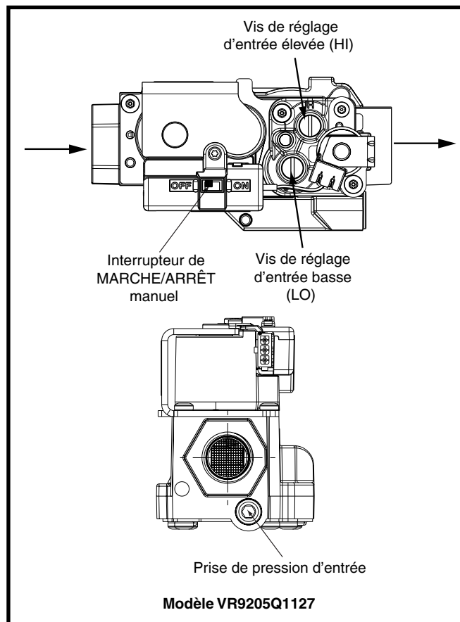
Figure 21. Vanne à gaz
